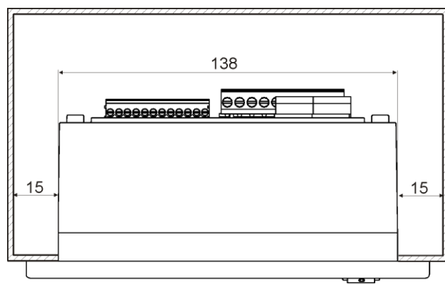
Рис. 10 Условия застройки регулятора
