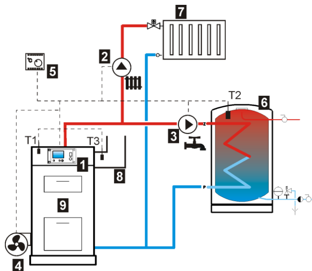
Рис. 6 Обслуживаемая регулятором гидравлическая схема, где: 1 – регулятор, 2 – насос центрального отопления, 3 – насос тёплой воды, 4 – вентилятор, 5 – комнатный термостат, 6 – бак тёплой воды, 7 – установка центрального отопления, 8 – дымоход, 9 – котёл, T1 – датчик температуры котла, T2 – датчик температуры тёплой воды, T3 – датчик температуры выхлопных газов (как опция, не требуется для нормальной работы).
