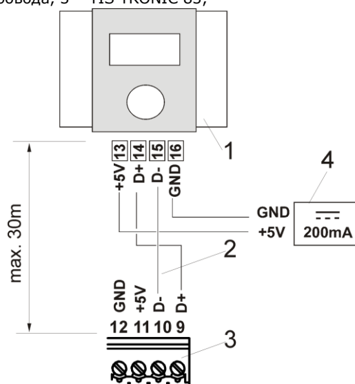
Рис. 15 Подключение комнатной панели TIS TRONIC 297 – двухпроводное, где: 1 – TIS TRONIC 297, 2 – провода, 3 – TIS TRONIC 83, 4 – блок питания 5В мин 200мА.
