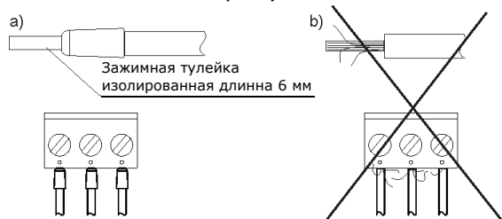
Рис. 13 Страховка концов провода: а) правильная, б) неправильная
