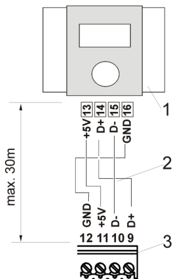
Рис. 14 Подключение комнатной панели TIS TRONIC 297 – четырёхпроводное, где: 1 – TIS TRONIC 297, 2 – провода, 3 – TIS TRONIC 83,
