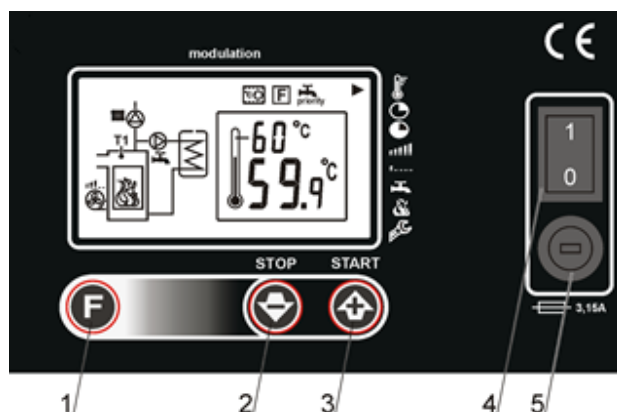
Рис. 1 Вид клавиатуры
