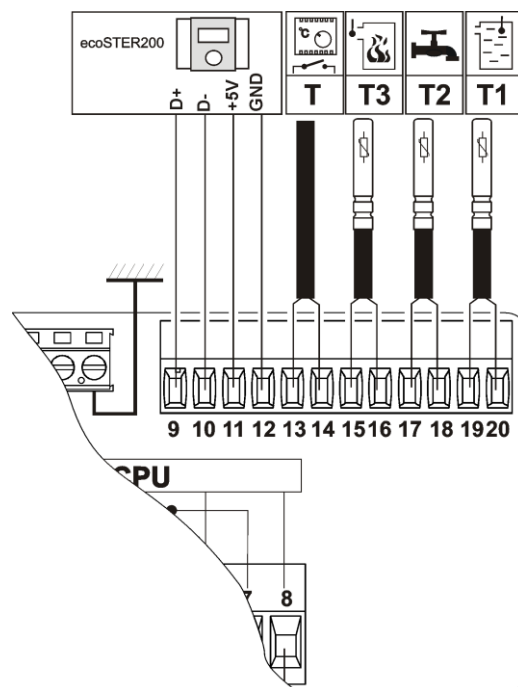
Рис. 12 Схема электрических соединений с внешними устройствами, версия ES.
