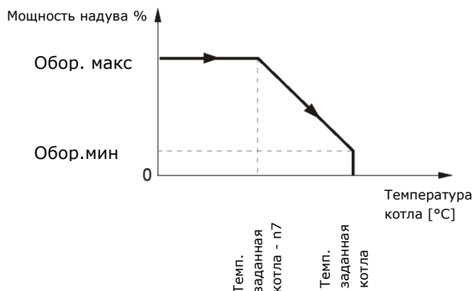
Рис. 17 Снижение оборотов вентилятора при классической регуляции
