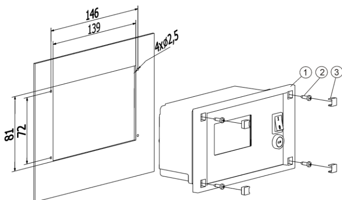
Рис. 8 Установка регулятора в монтажной доске, где: 1 - регулятор, 2 - винт 2.9х9, 3 - заглушка.
