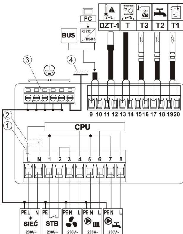
Рис. 11 Схема электрических соединений с внешними устройствами, версия ST. где: T1 – датчик температуры котла (тип CT4), T2 – датчики температуры тёплой воды (тип CT4), T3 – датчик температуры выхлопных газов (тип CT2s, CT2s-2), T – комнатный термостат, DZT-1 – дополнительная термическая страховка (тип DZT-1 85°C или 90°C), RS232/RS485 –преобразователь, BUS – соединение цифровой коммуникации с компьютером (опция), 1 – сетевой предохранитель в регуляторе, 2 – сетевой выключатель в регуляторе, 3 – охранные зажимы PE, 4 – металлический корпус регулятора, СЕТЬ – сетевой провод, STB – ограничитель температуры безопасности,
