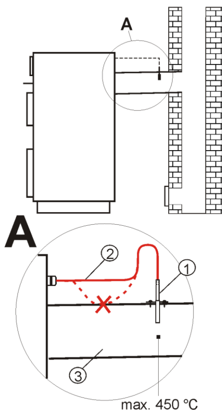
Рис. 16 Подключение датчика выхлопных газов, где: 1 – датчик температуры выхлопных газов СТ2s-2, 2 – провод датчика, 3 – дымоход.
